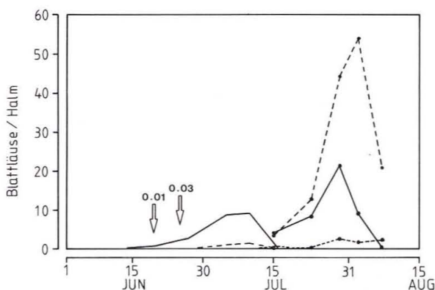
Abb. 2.2.5: Verlauf der Populationsdynamik der Getreideblattläuse im Feld und in Isolationskäfigen im Jahr 1985. — M. dirhodum im Feld, ●—● M. dirhodum im Käfig, - - - S. avenae im Feld, ●- - - S. avenae im Käfig, ····· verpilzte Blattläuse.
