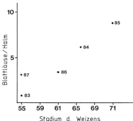
Abb. 2.2.1: Beziehung zwischen der Maximaldichte der Getreideblattläuse in den Jahren 1983 bis 1987 und dem Entwicklungsstadium des Weizens, auf dem sie erreicht wurde.
