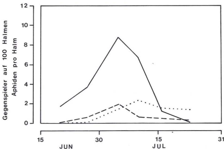
Abb. 2.2.4: Abundanz der aus Blattlausmumien geschlüpften Primärparasitoiden und Hyperparasitoiden. Nicht-insektizidbehandelte Parzellen des Feldversuchs 1985. — Summe Aphiden, - - - Aphidiidae, ..... Hyperparasitoide.
