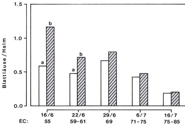
Abb. 2.2.7: Einfluß der Pflanzenbauintensität auf die Populationsdichte der Getreideblattläuse, Feldversuch 1983. Leere Säulen: Sorte 'Jubilar' mit 120 kg N/ha gedüngt; schraffierte Säulen: Sorte 'Okapi' mit 180 kg N/ha gedüngt. Mit unterschiedlichen Buchstaben gekennzeichnete Säulen eines Erhebungstermins sind signifikant voneinander verschieden.
