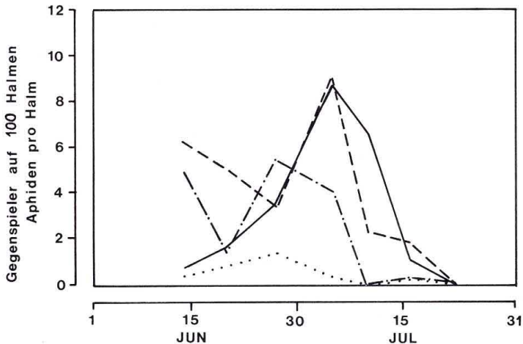
Abb. 2.2.3: Eiablage stenophager Blattlausfeinde auf nicht-insektizidbehandelten Parzellen des Feldversuchs 1985. — Summe Aphiden, ---- Syrphideneier, - - - - Coccinellideneier, ..... Chrysopideneier.
