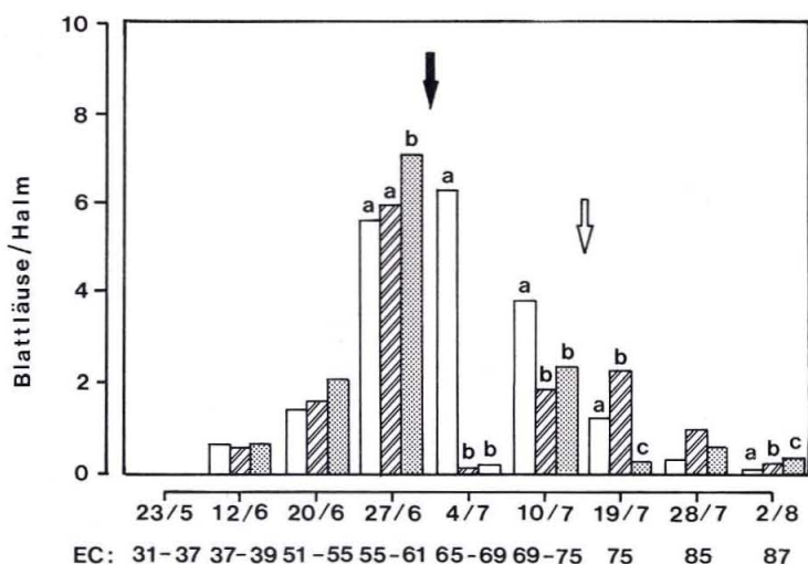
Abb. 2.2.8: Einfluß der Pflanzenschutzintensität auf die Populationsdynamik der Getreideblattläuse, Feldversuch 1984. Leere Säulen: Intensitätsstufe 1, schraffierte Säulen: Intensitätsstufe 2, gepunktete Säulen: Intensitätsstufen 3 (vgl. Abschn. Methodik). Ausgefüllter Pfeil: Einsatz von 0,3 kg/ha Pirimor in den Stufen 2 und 3, leerer Pfeil: Einsatz von 0,3 kg/ha Pirimor nur in der Stufe 3. Mit unterschiedlichen Buchstaben gekennzeichnete Säulen eines Erhebungstermins sind signifikant voneinander verschieden.
