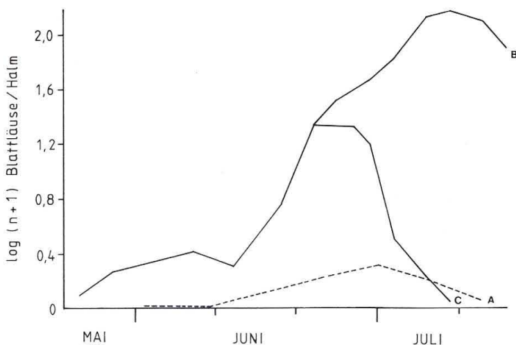
Abb. 2.2.6: Populationsdynamik von M. dirhodum während des Isolationsversuchs 1986 im Feld (Kurve A) und in Isolationskäfigen (Kurven B + C). Ein Teil der Experimentalpopulationen war nach dem Abdecken der Käfige dem Angriff natürlicher Feinde ausgesetzt (Kurve C). Logarithmischer Maßstab (weitere Erläuterungen siehe Text) (nach Becker 1987).
