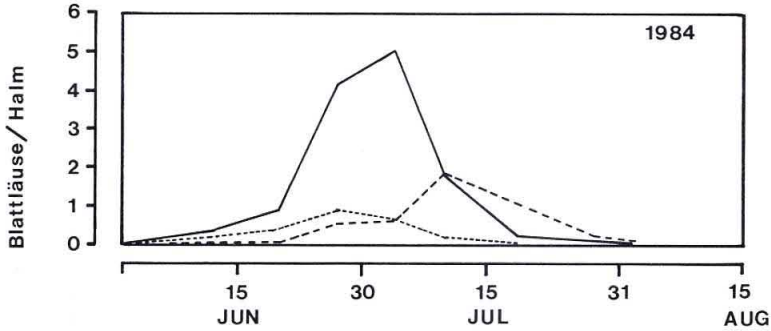
Abb. 2.2.2: Populationsdynamik der Getreideblattläuse im Jahr 1984. — Metopolophium dirhodum , ---- Sitobion avenae , - - - - Rhopalosiphum padi .
