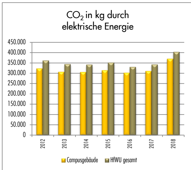
Abb. 50: CO 2 durch elektrische Energie
